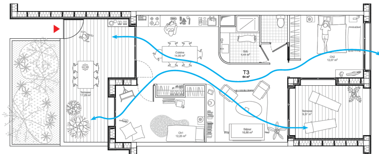
Plan de logement T3 en rdc sur cour jardin
